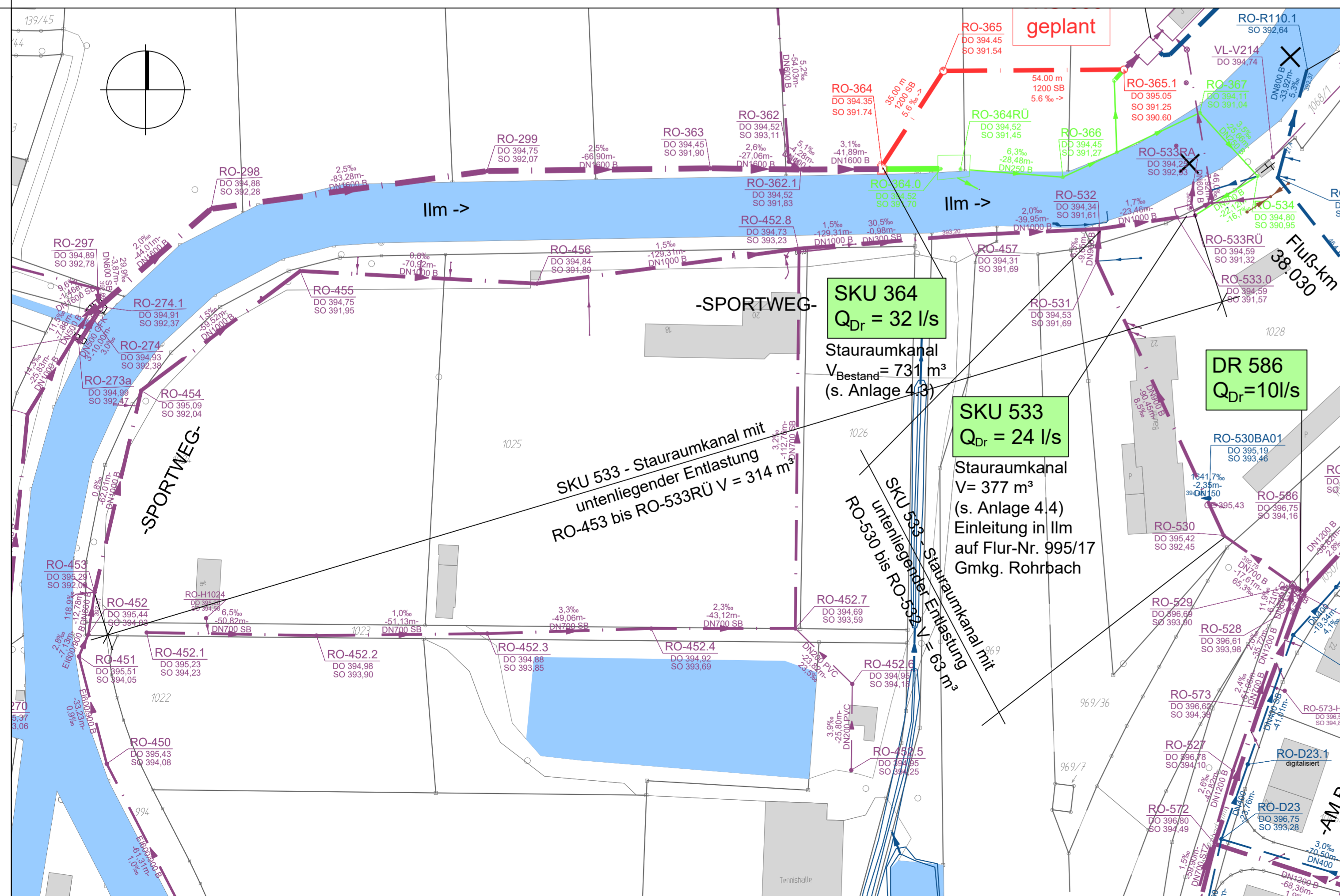
Lageplan M=1:1000
