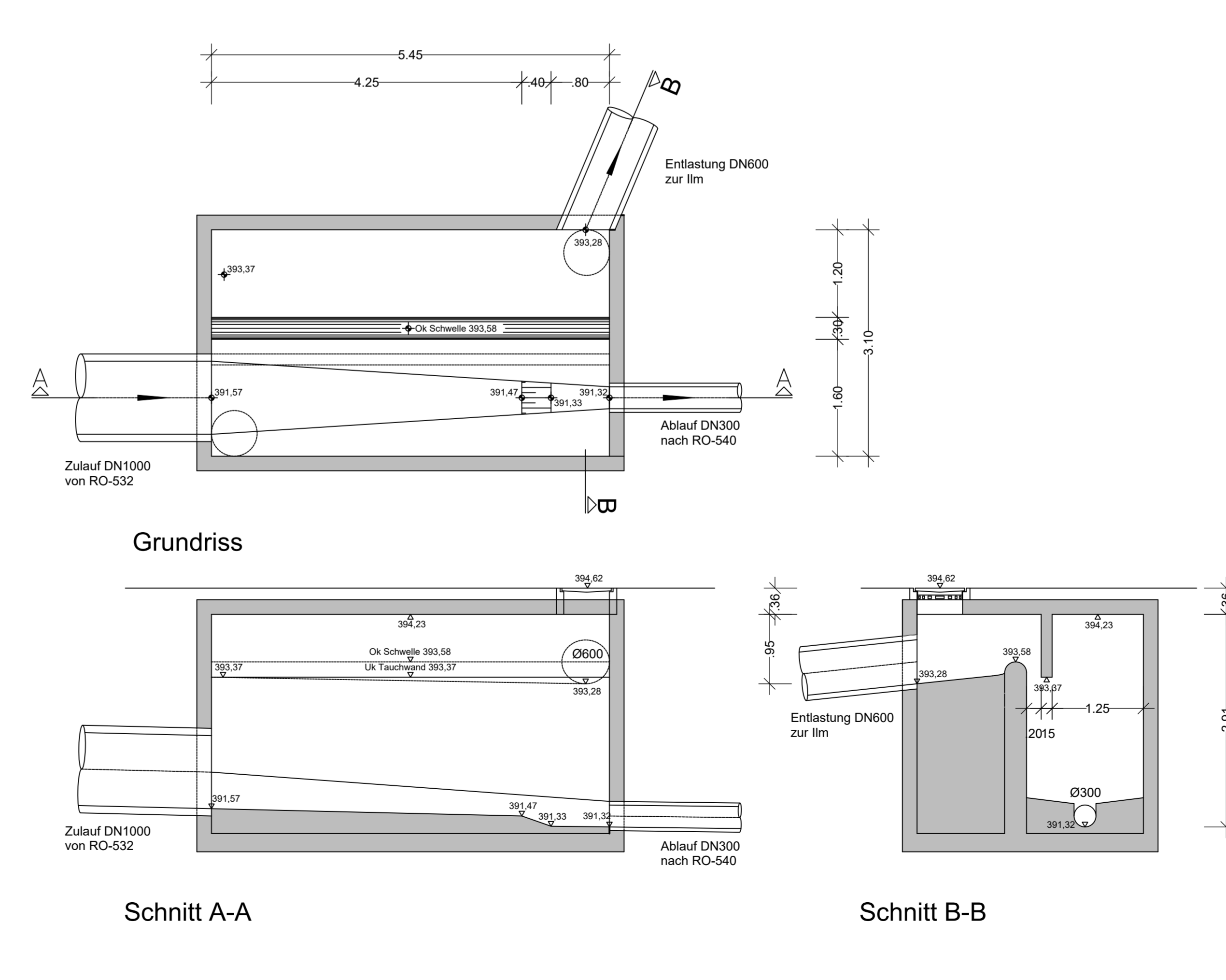
Trennbauwerk M=1:50 (RO-533RÜ)
