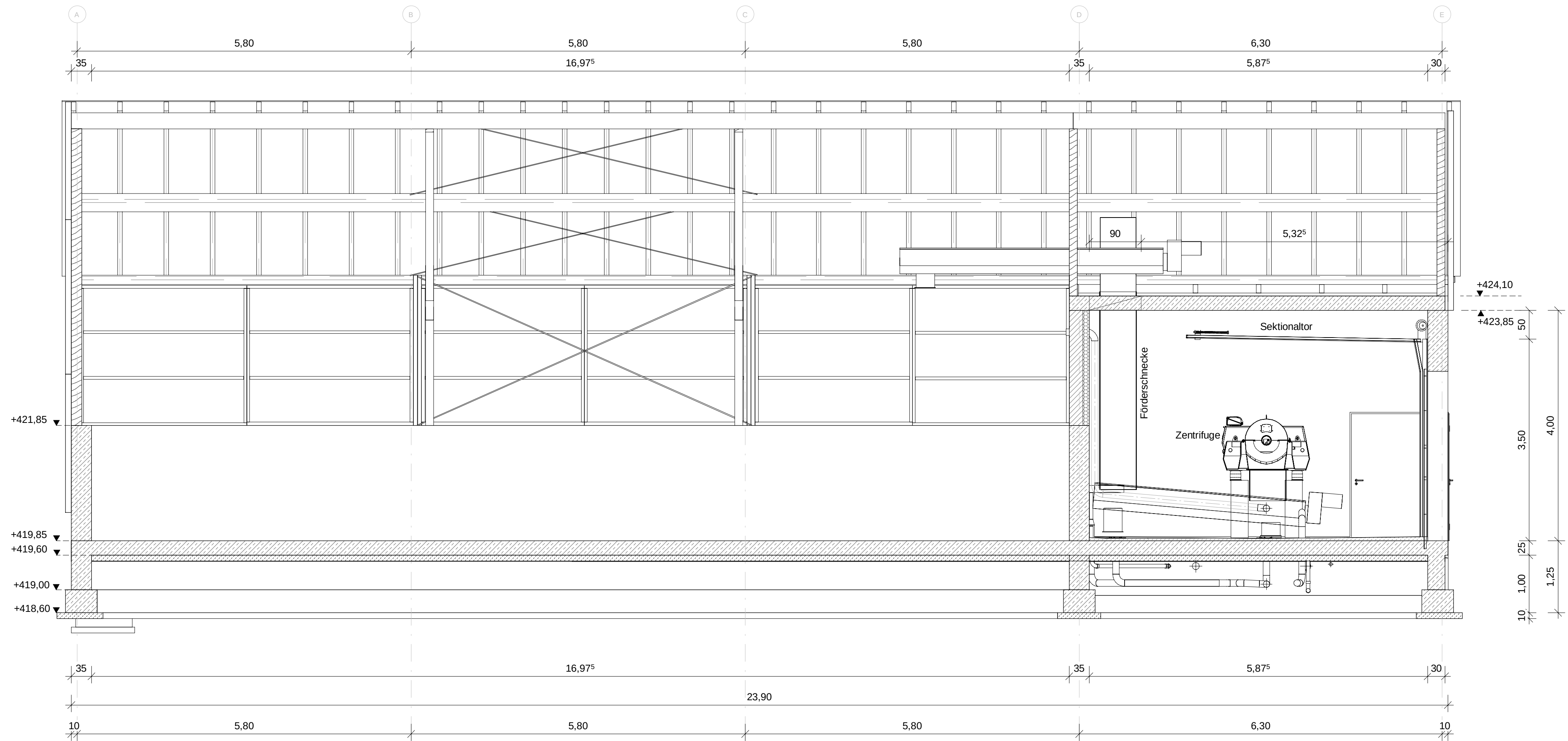
SCHNITT A-A
