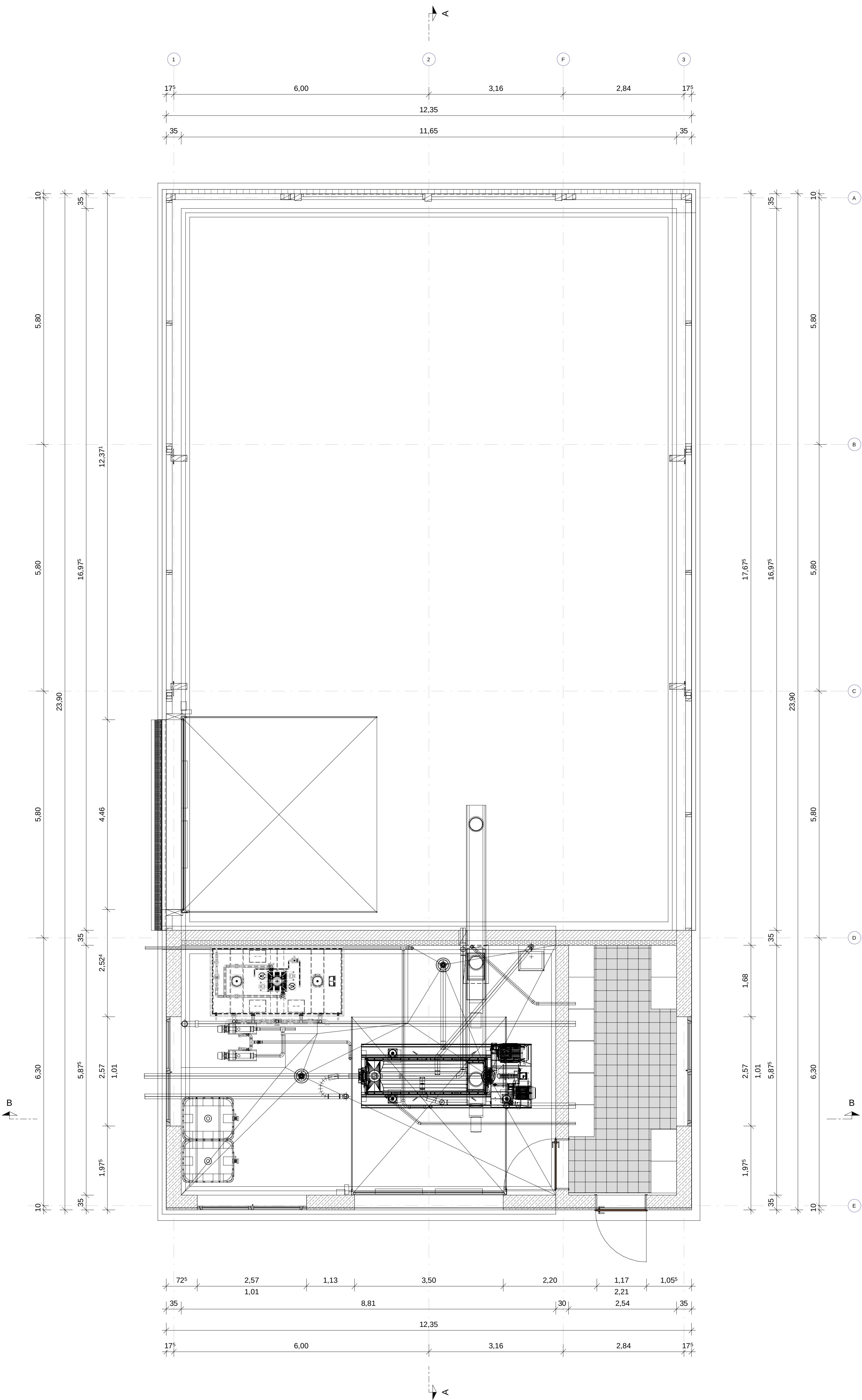
GRUNDRISS
