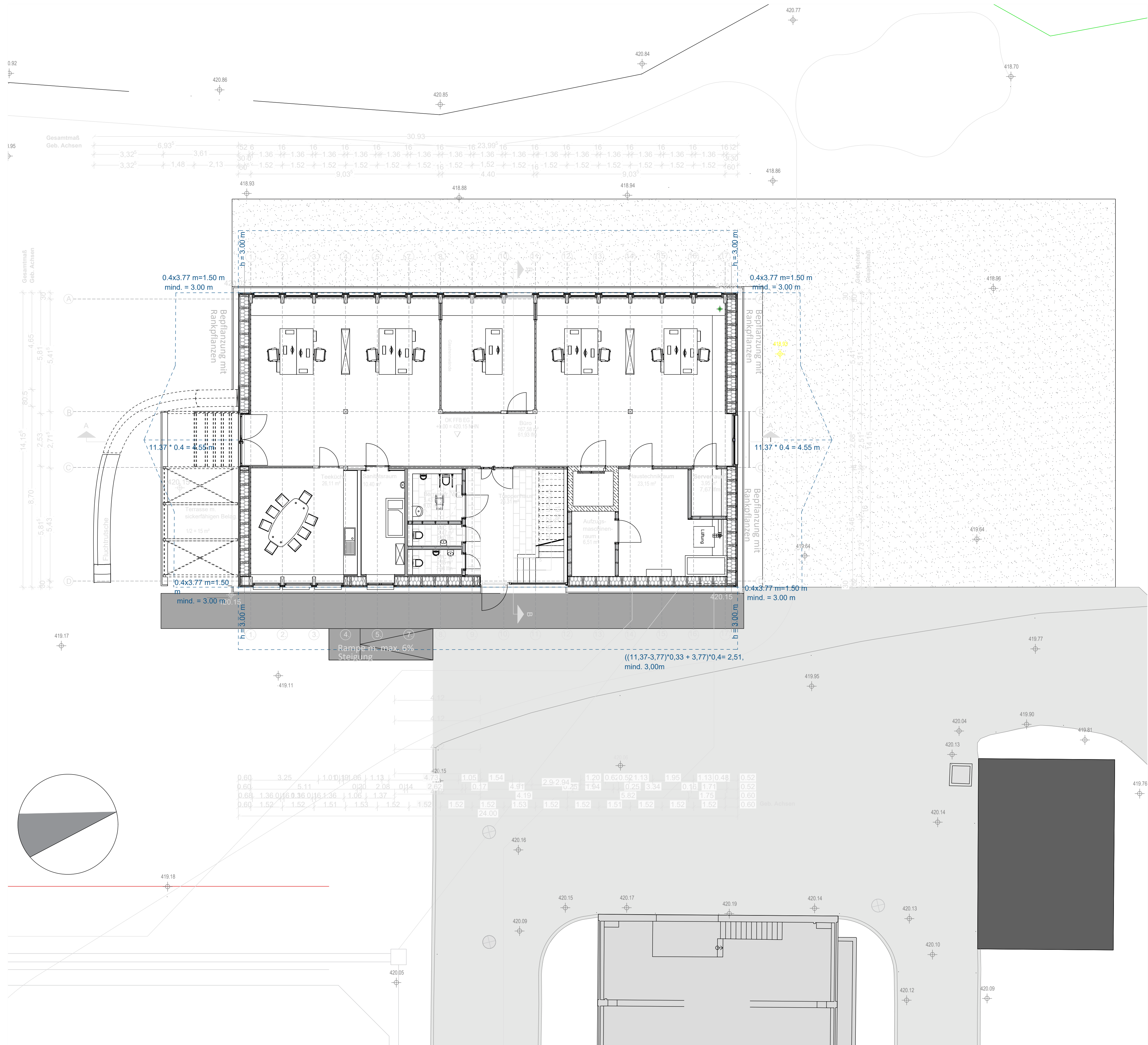
Grundriss Erdgeschoss
