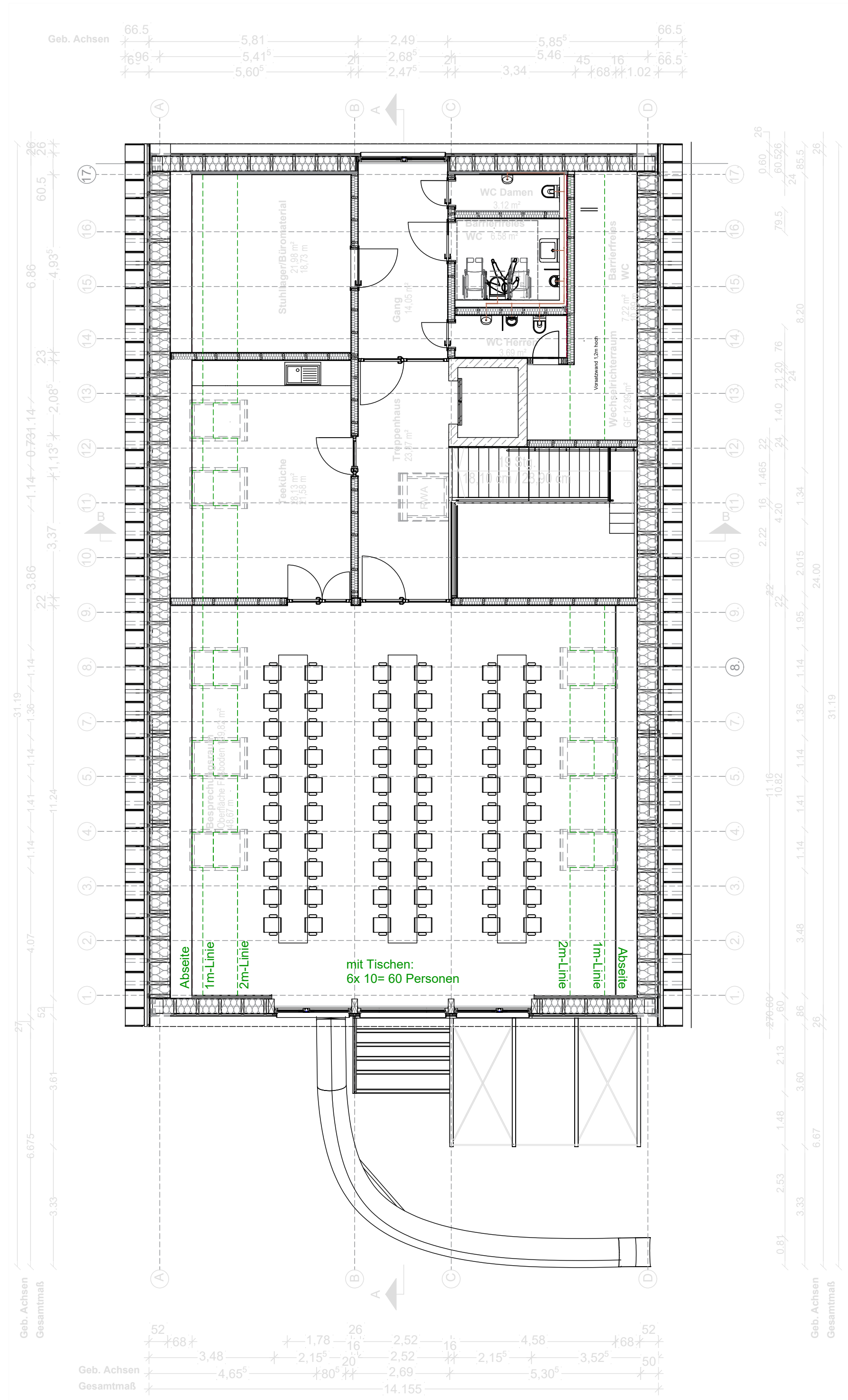
Grundriss Dachgeschoss
