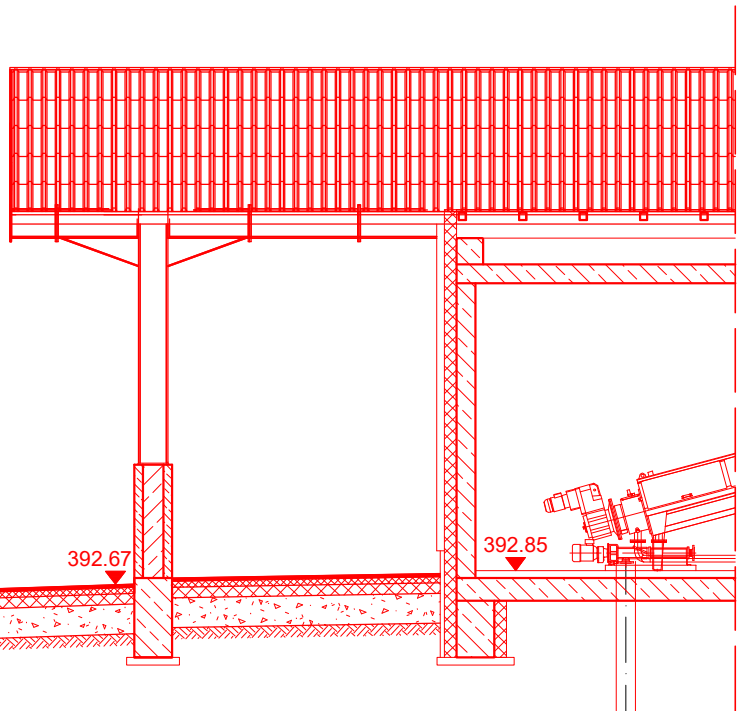
Schlammwässerung
