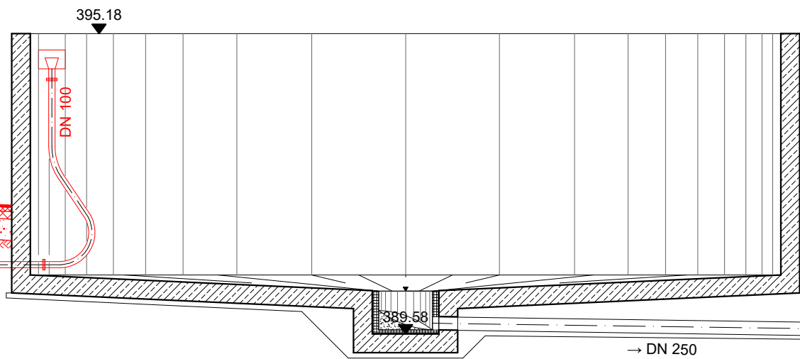
Vorhaltebecken
