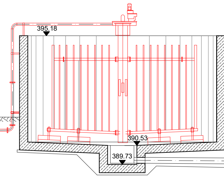
Voreindicker
