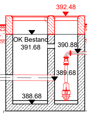
Vorschacht
