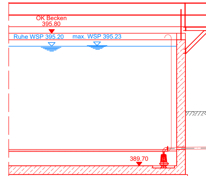
SU-Becken 2
