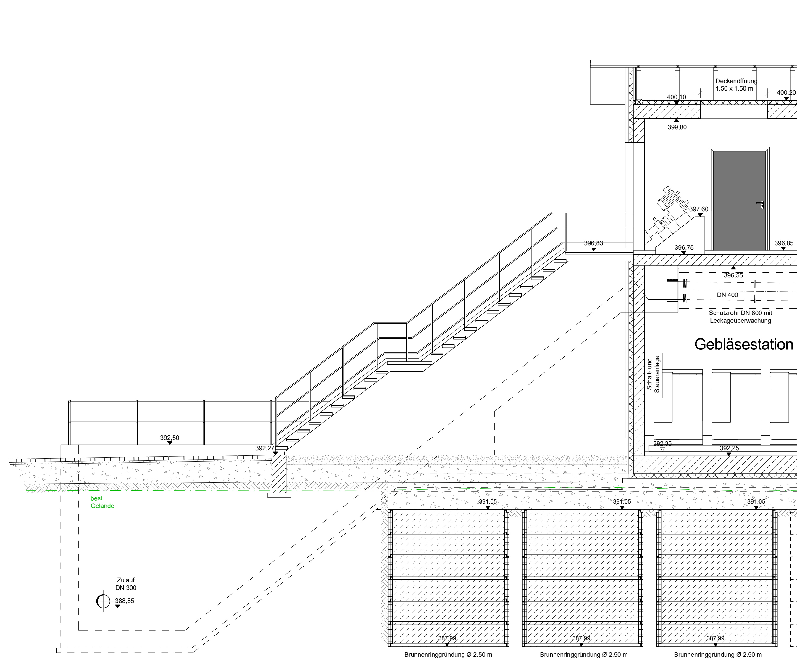
Schnitt C - C
