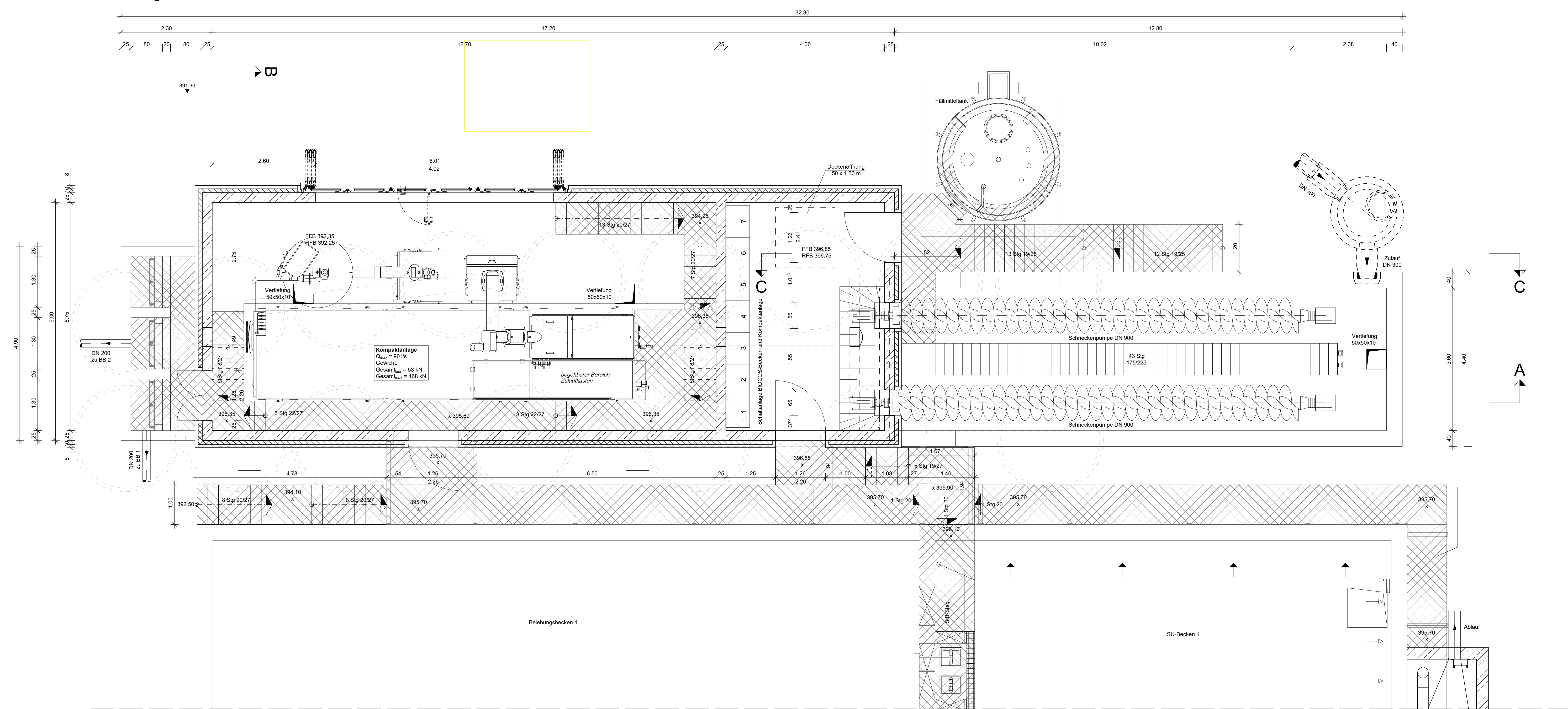
Grundriss Obergeschoss
