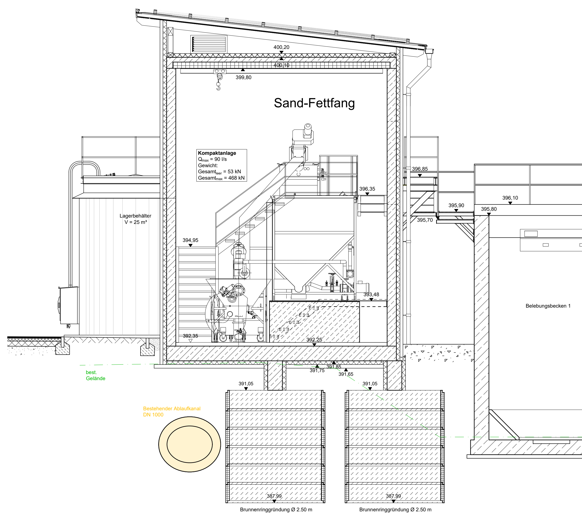
Schnitt B - B
