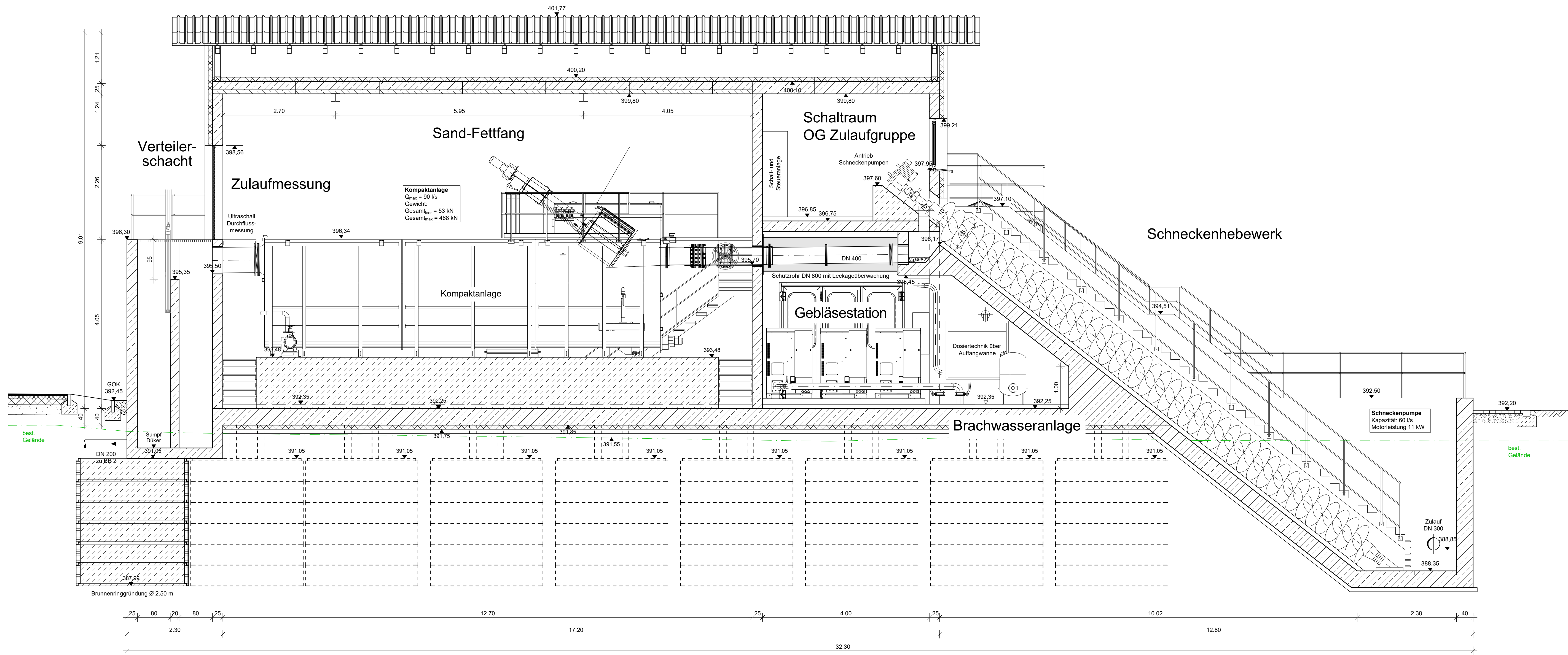
Schnitt A - A
